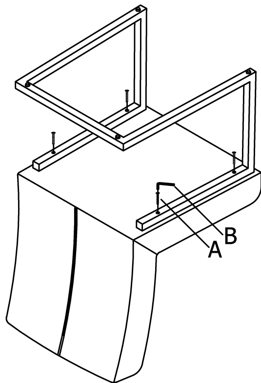
STEP1/ÉTAPE1
