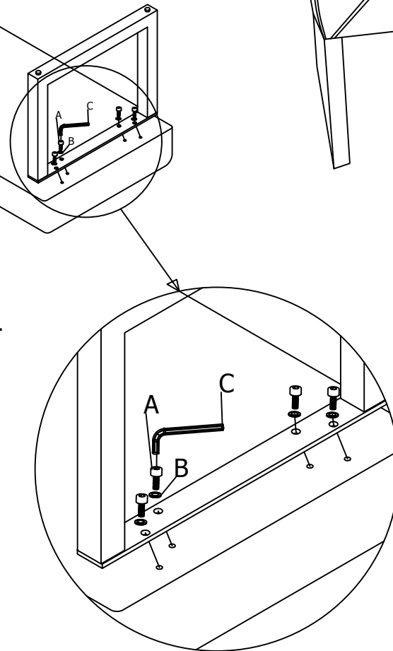
STEP1 ÉTAPE1
